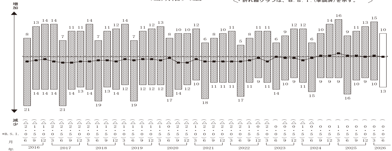
短期借入金
